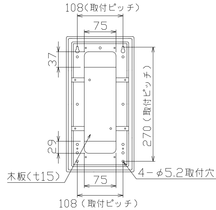
配線孔寸法図(////部開口)
