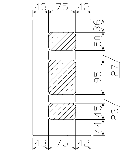
配線孔寸法図(////部開口)
